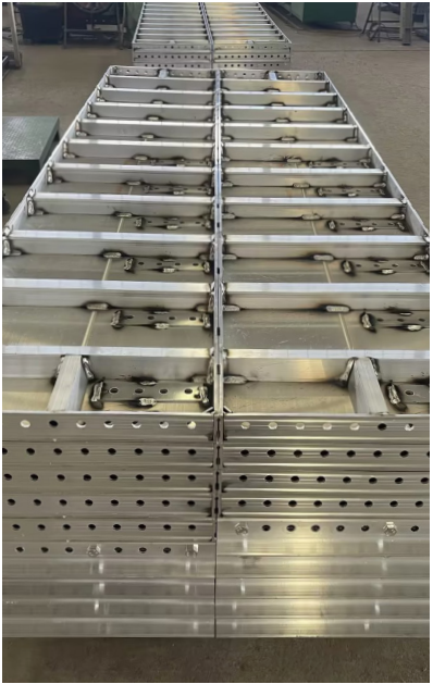
Formwork Example / 模板实例图
